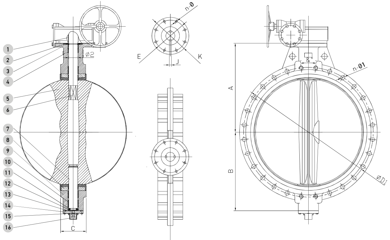
FIG. 4 DN700-1200
