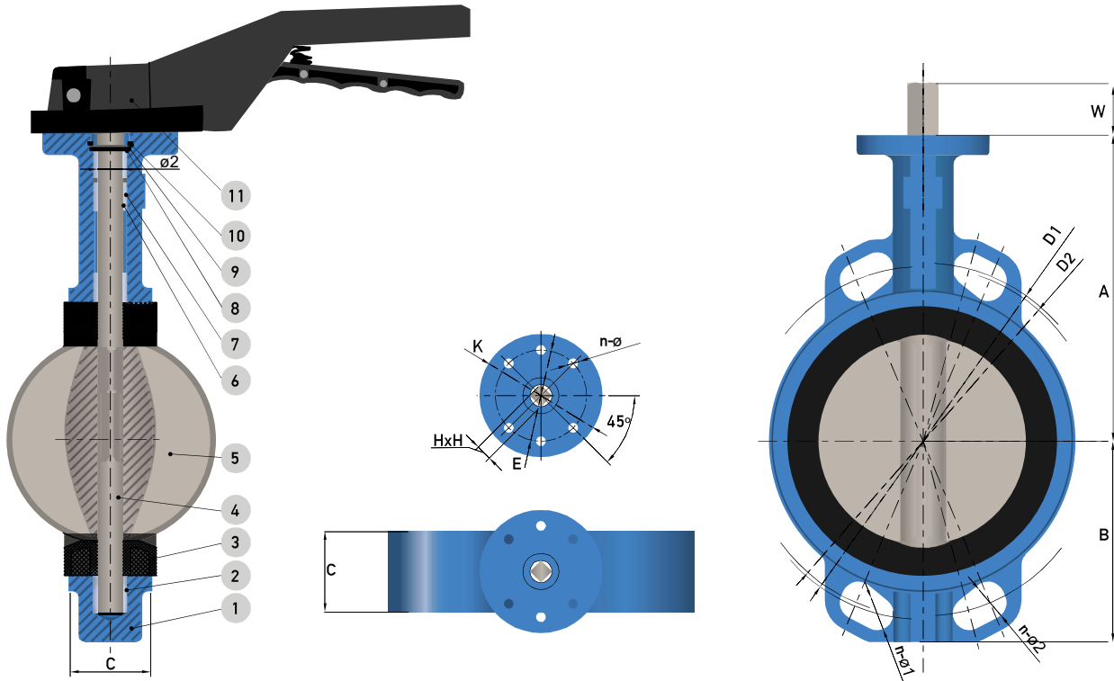
FIG. 1 DN40-200
