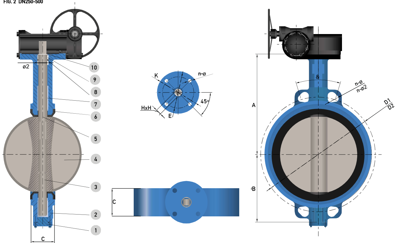
FIG. 2 DN250-500
